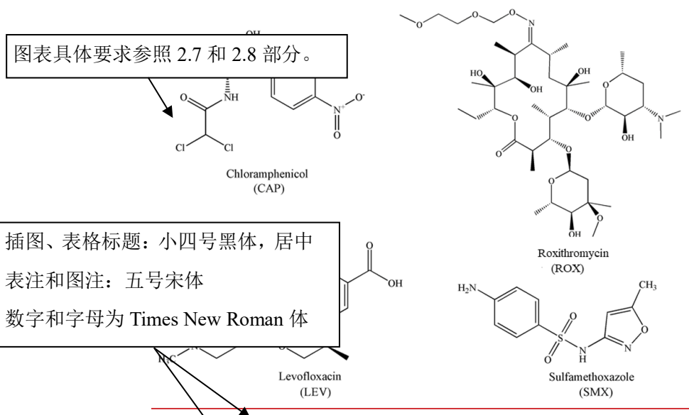
图 1.1 四种抗生素的化学结构式
